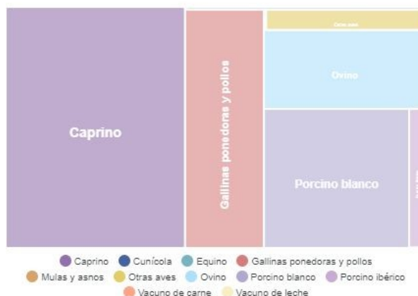
Gráfico 56: Número de cabezas y emisiones por categoría de ganado en Levante III.1 (2021). Fuente: Huella de Carbono Municipal. Junta de Andalucía.
