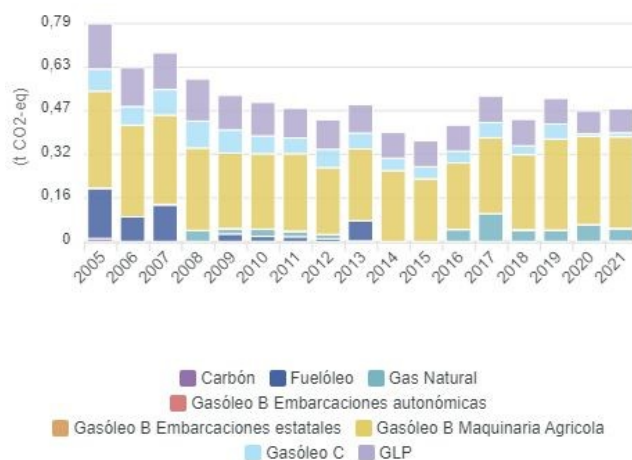
Gráfico 50: Evolución de emisiones GEI per cápita por año y tipo de combustible - inst fijas en Levante III.1 (2005-2021). Fuente: Huella de Carbono Municipal. Junta de Andalucía.
