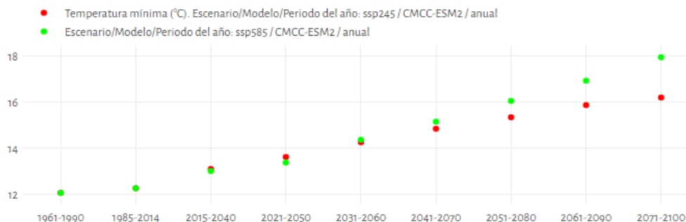
Ilustración 12: Evolución de las temperaturas mínimas anuales en los diferentes periodos.
