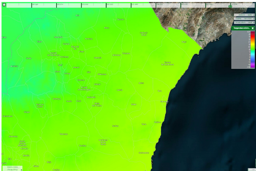
Ilustración 54: Evolución de las temperaturas mínimas anuales en el periodo comparado 2071-2100. Fuente: SICMA
