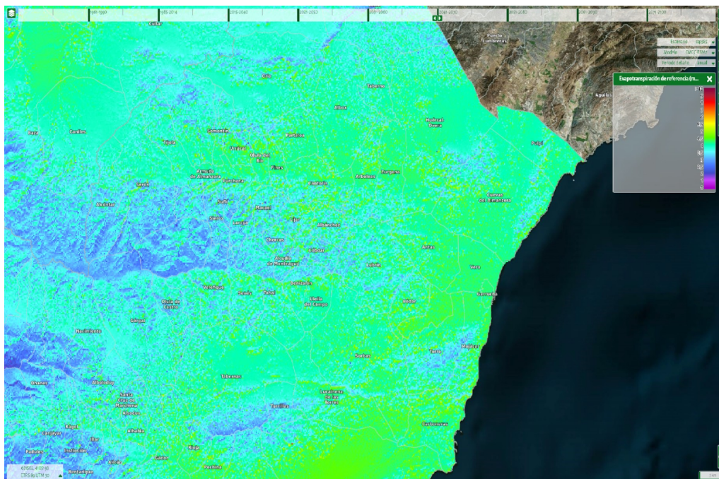
Ilustración 49: Evolución de la Evapotranspiración de referencia en el periodo comparado 2041-2070. Fuente: SICMA
