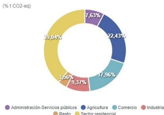
Gráfico 46: Porcentaje de emisiones por consumo eléctrico por subsectores en Levante III.1 (2021). Fuente: Huella de Carbono Municipal. Junta de Andalucía.
