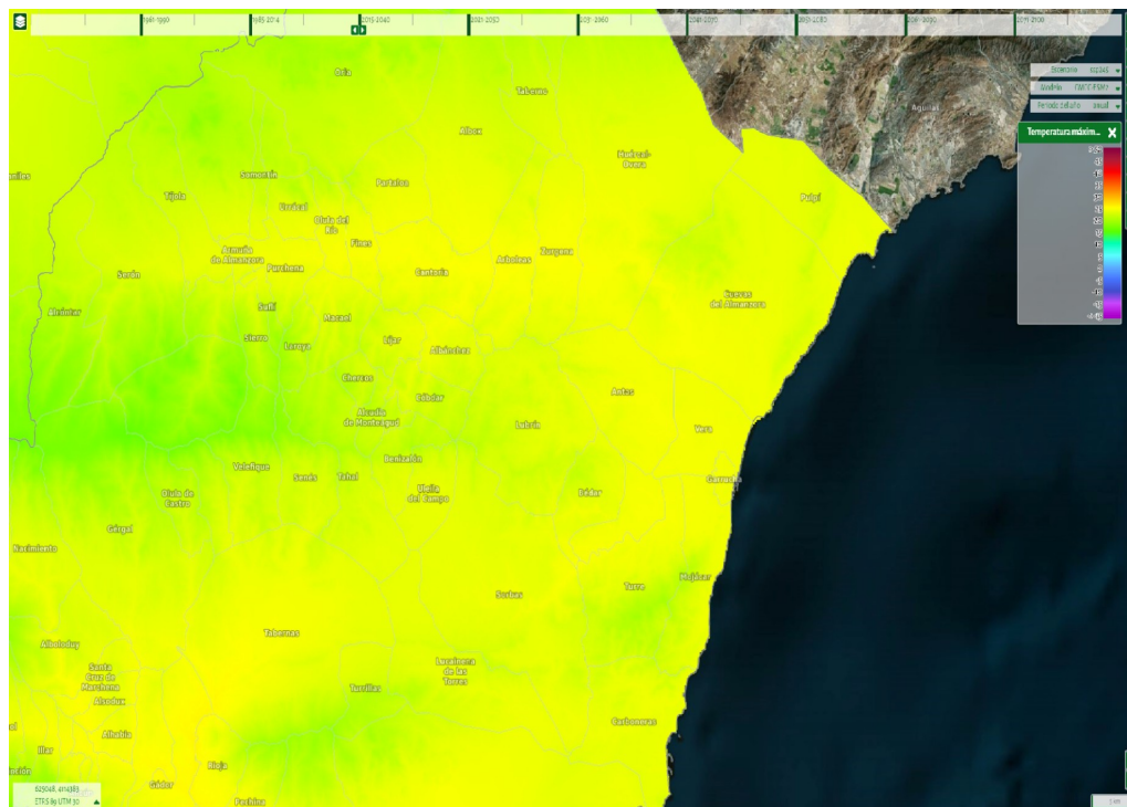
Ilustración 18: Evolución de las temperaturas máxima anual en el periodo comparado
