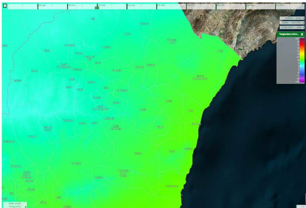
Ilustración 19: Evolución de las temperaturas mínimas anuales en el periodo comparado 2015-2040. Fuente: SICMA
