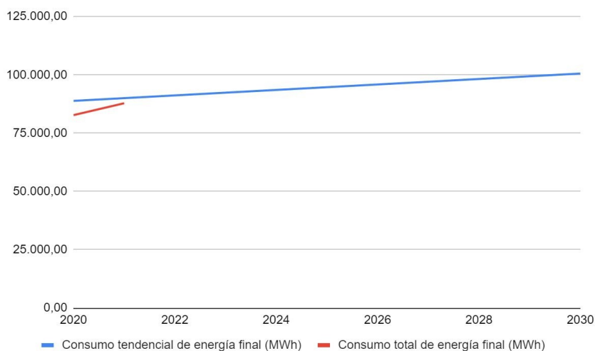
Gráfico 30: Evolución del consumo tendencial y del consumo de energía final (Mwh) en Sorbas (2020-2030). Fuente: Huella de Carbono Municipal. Junta de Andalucía.
