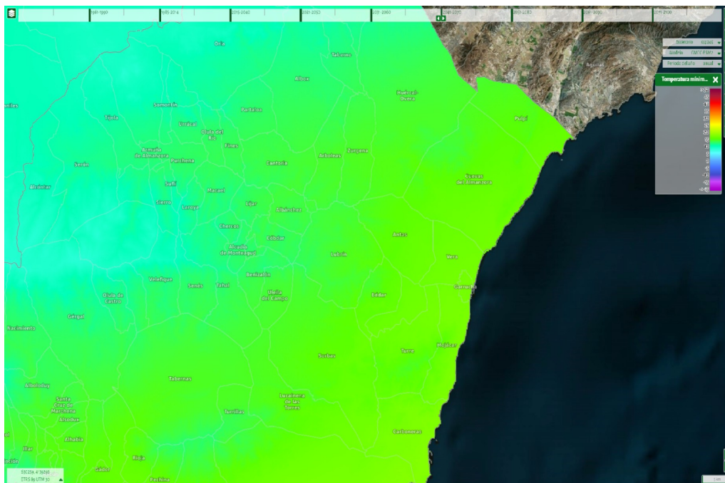
Ilustración 26: Evolución de las temperaturas mínimas anuales en el periodo comparado 2041-2070. Fuente: SICMA
