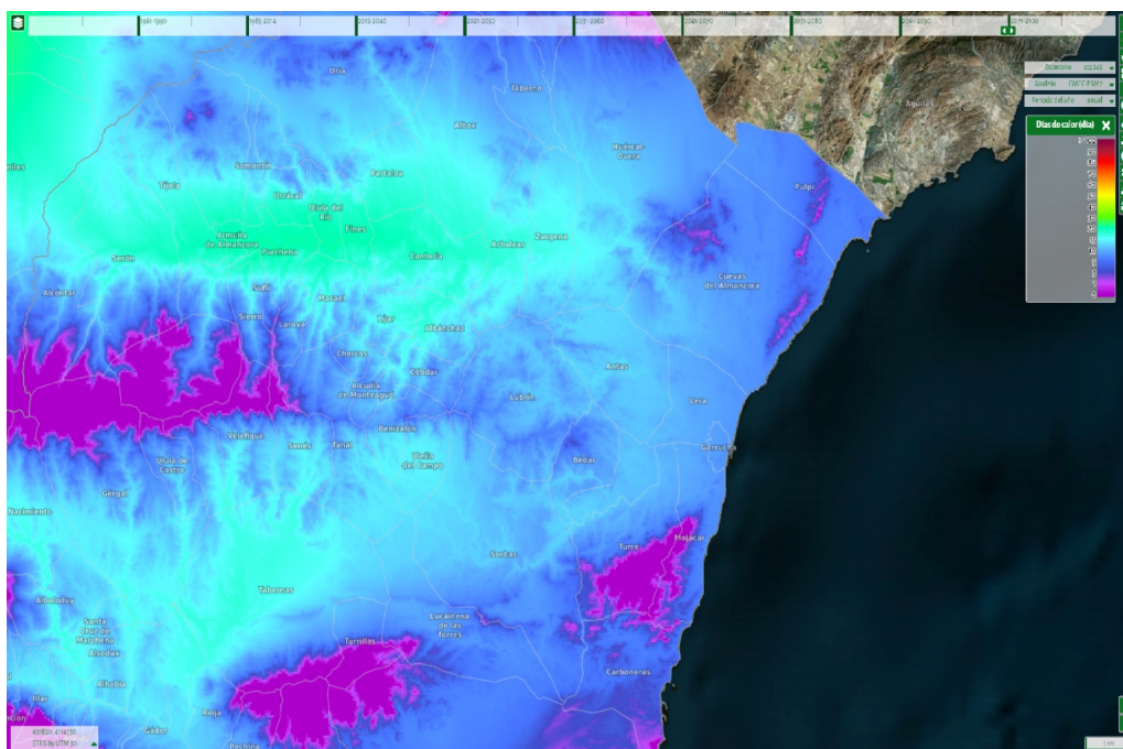
Ilustración 87: Evolución del número de días de calor (40 °C) en el periodo comparado 2071-2100. Fuente: SICMA
