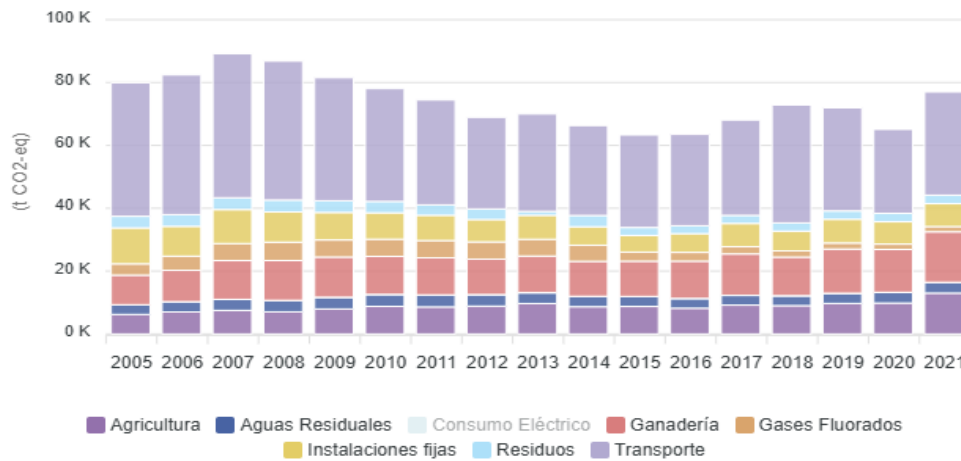
Gráfico 43: Evolución de emisiones difusas, por año y sector en Levante III.1 (2005-2021). Fuente: Huella de Carbono Municipal. Junta de Andalucía.
