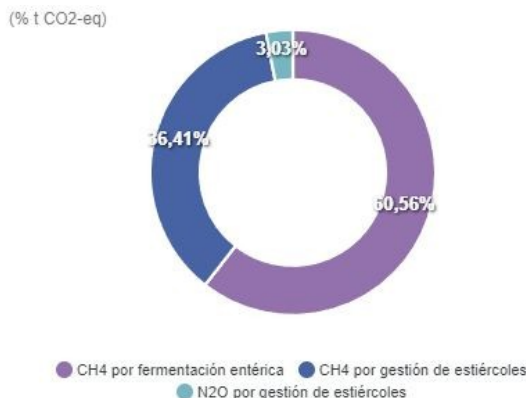
Gráfico 55: Porcentaje según el tipo de emisiones – ganadería en Levante III.1 (2021). Fuente: Huella de Carbono Municipal. Junta de Andalucía.
