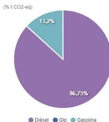
Gráfico 13: Emisiones por tipo de combustible en Sorbas (2021). Fuente: Huella de Carbono Municipal. Junta de Andalucía.
