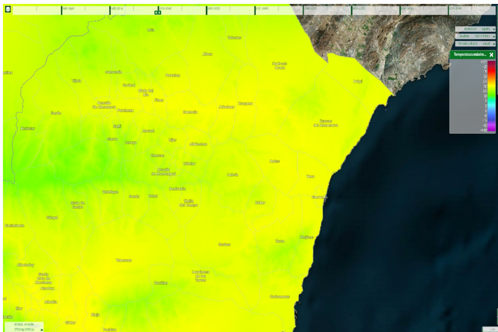
Ilustración 39: Evolución de las temperaturas máximas anuales en el período comparado 2015-2040. Fuente: SICMA
