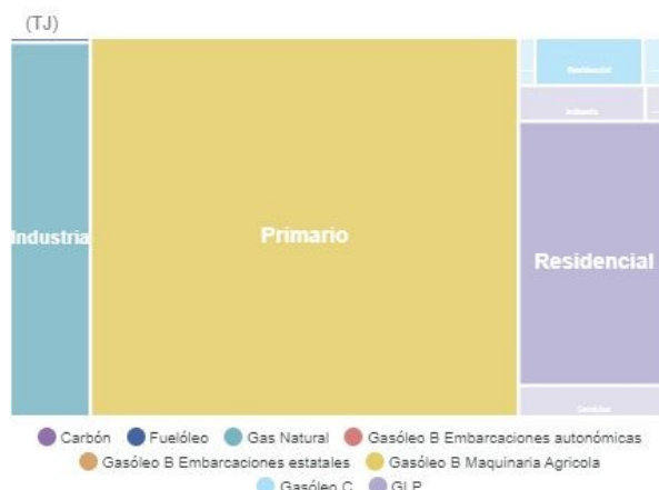
Gráfico 64: Consumo de combustibles fósiles en instalaciones fijas per cápita por tipo y sector en Levante III.1 (2021). Fuente: Huella de Carbono Municipal. Junta de Andalucía.
