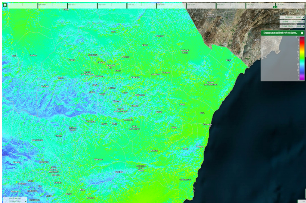
Ilustración 35: Evolución de la evapotranspiración de referencia en el periodo comparado 2071-2100. Fuente: SICMA
