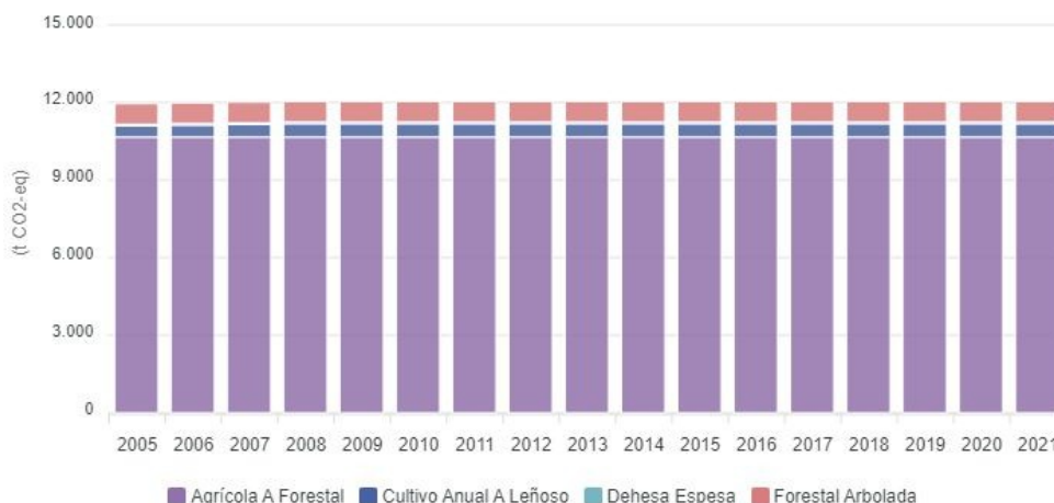
Gráfico 61: Evolución de absorciones GEI por año y tipo de actividad – Sumidero en Levante III.1 (2005-2021). Fuente: Huella de Carbono Municipal. Junta de Andalucía.
