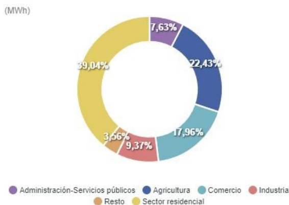
Gráfico 63: Consumo eléctrico por subsectores en Levante III.1 (2021).
