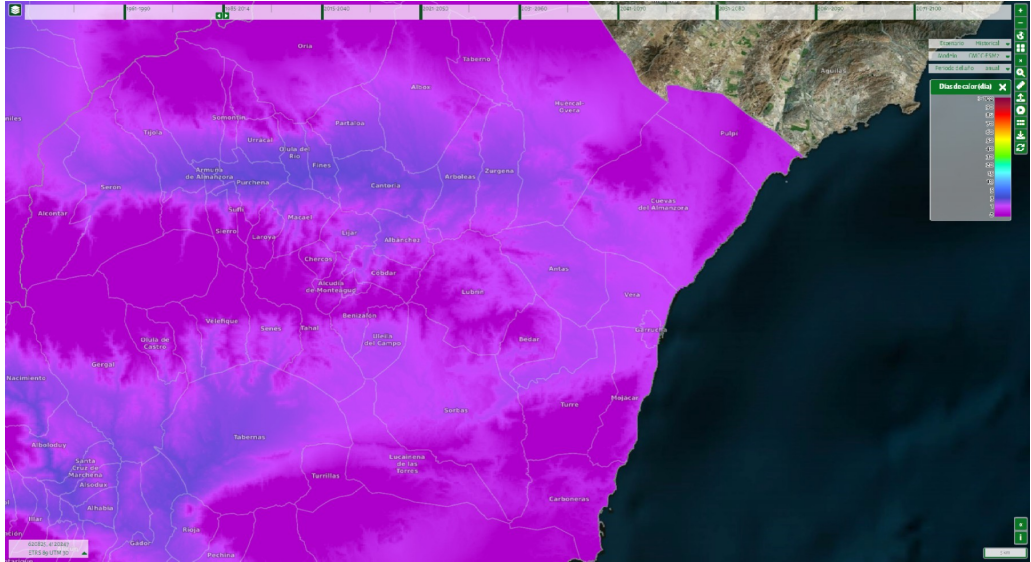
Ilustración 66: Evolución del número de días de calor (40 °C) de tendencia histórica. Fuente: SICMA
