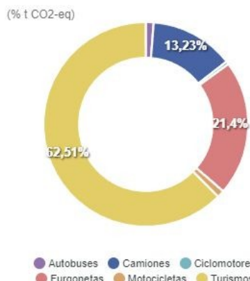
Gráfico 48: Porcentaje de emisiones por tipo de vehículo en Levante III.1 (2021). Fuente: Huella de Carbono Municipal. Junta de Andalucía.
