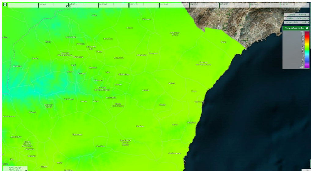
Ilustración 3: Evolución de las temperaturas medias anuales de tendencia histórica.
