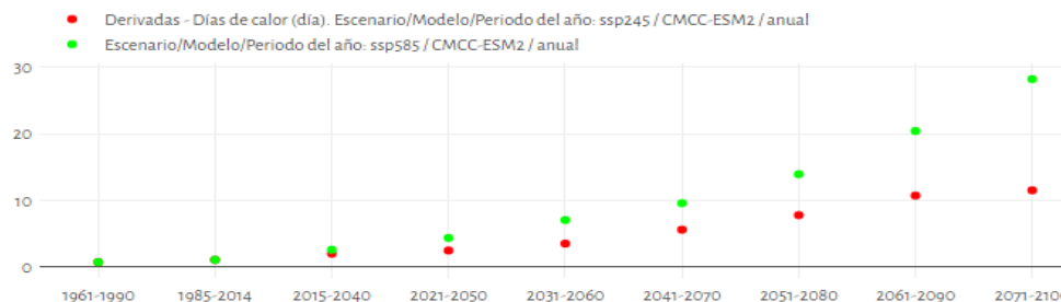
Ilustración 15: Evolución de los días de calor anuales en los diferentes periodos.
