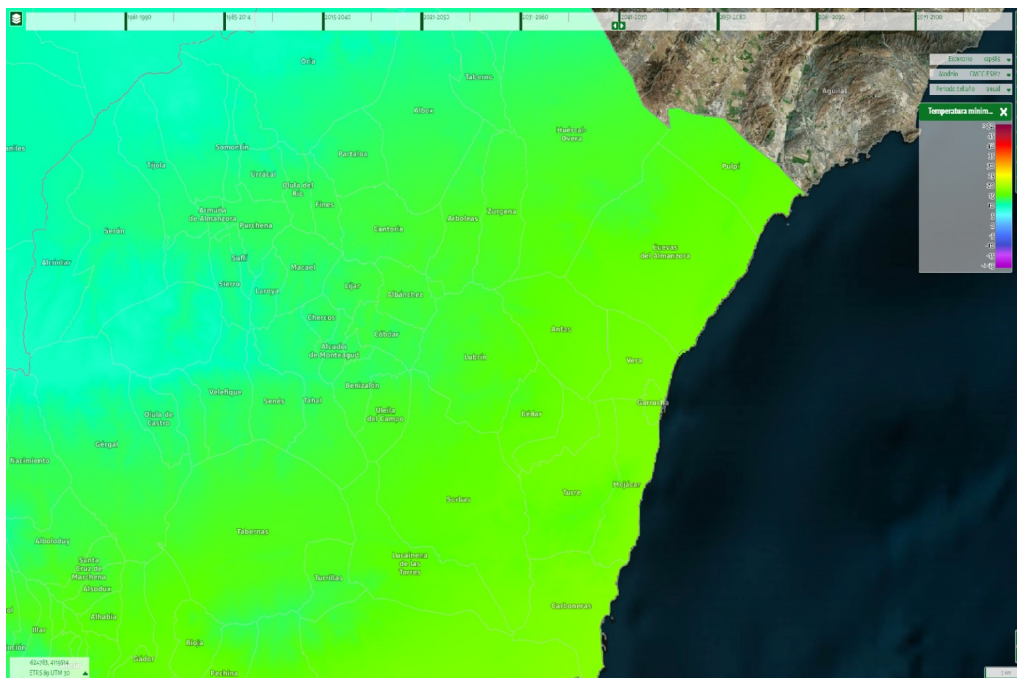
Ilustración 47: Evolución de las temperaturas mínimas anuales en el periodo comparado 2041-2070. Fuente: SICMA
