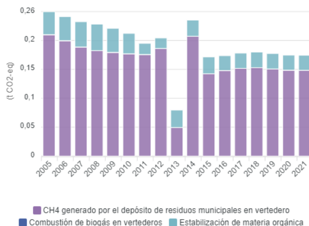
Gráfico 52: Evolución de emisiones GEI per cápita por residuos en Levante III.1 (2005-2021). Fuente: Huella de Carbono Municipal. Junta de Andalucía.
