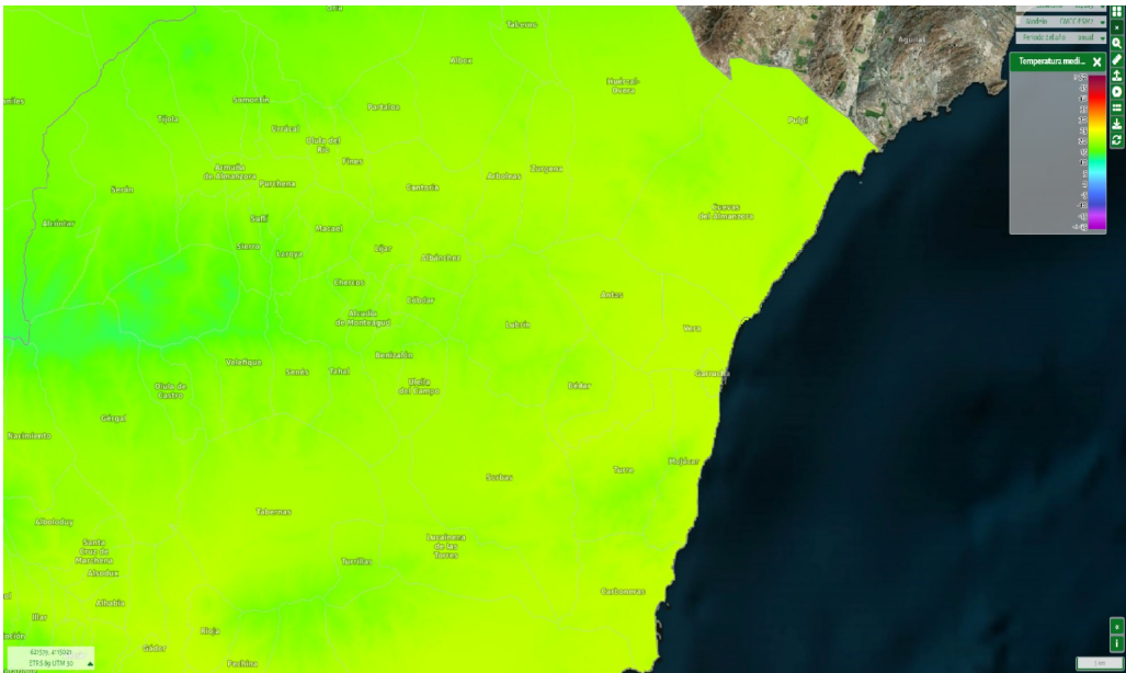
Ilustración 75: Evolución de las temperaturas medias anuales en el periodo comparado 2041-2070. Fuente: SICMA
