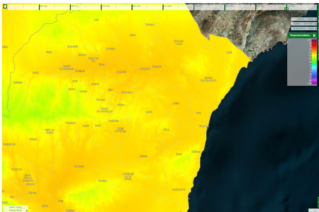
Ilustración 83: Evolución de las temperaturas máximas anuales en el periodo comparado 2071-2100. Fuente: SICMA
