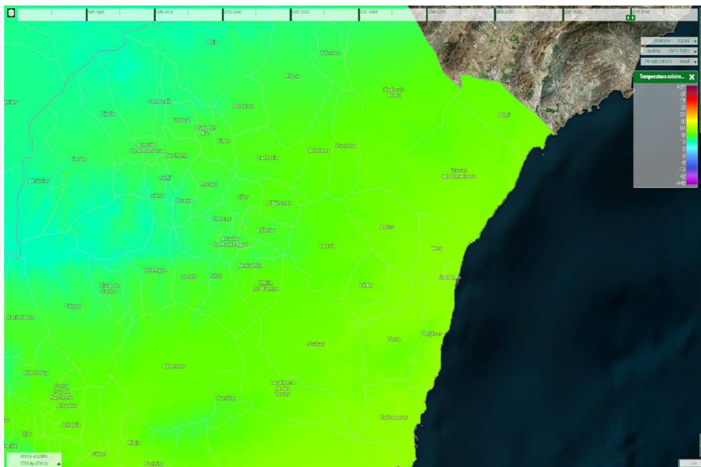
Ilustración 33: Evolución de la temperatura mínima anual en el periodo comparado 2071-2100. Fuente: SICMA
