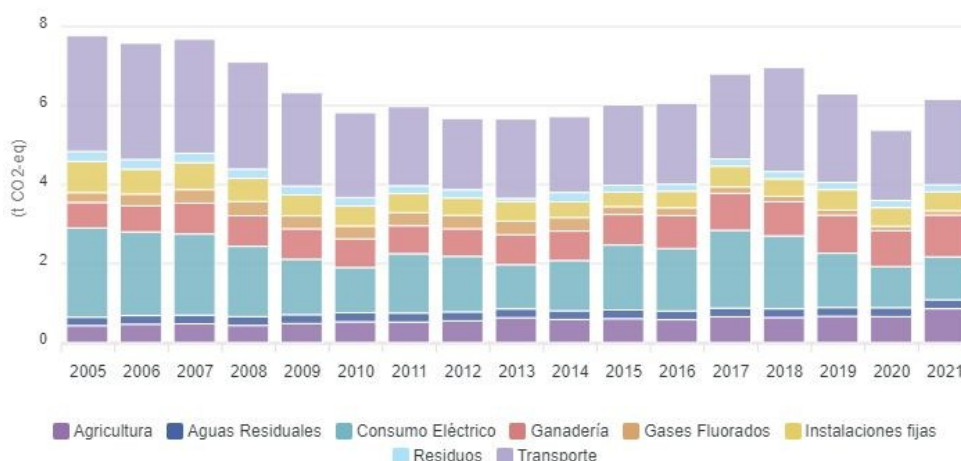
Gráfico 41: Evolución de emisiones GEI per cápita, por año y sector en Levante III.1 (2005-2021). Fuente: Huella de Carbono Municipal. Junta de Andalucía.
