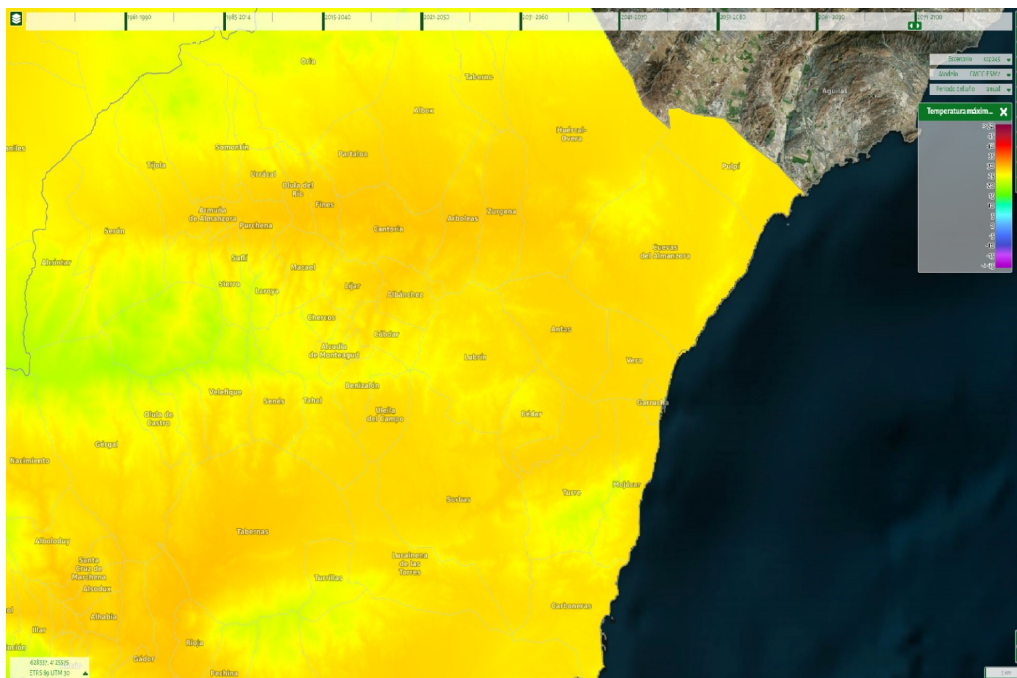
Ilustración 32: Evolución de las temperaturas máximas anuales en el período comparado 2071-2100. Fuente: SICMA
