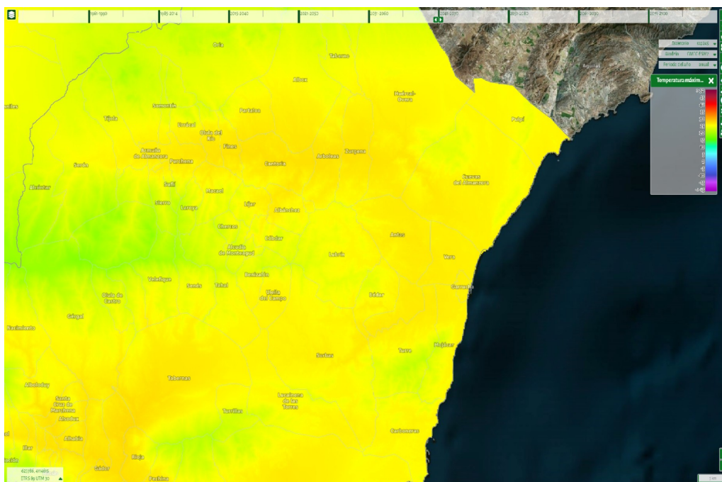
Ilustración 76: Evolución de las temperaturas máximas anuales en el periodo comparado 2041-2070. Fuente: SICMA
