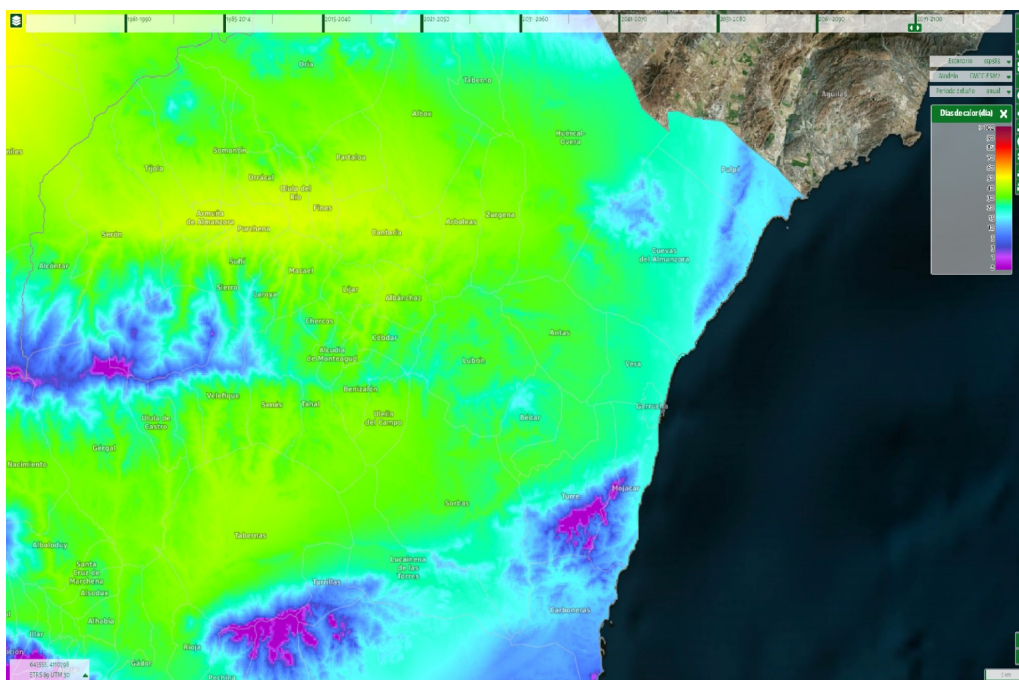
Ilustración 108: Evolución del número de días de calor (40 °C) en el periodo comparado 2071-2100. Fuente: SICMA
