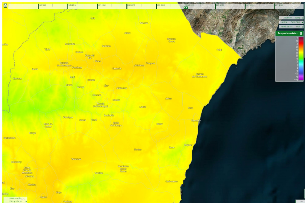
Ilustración 46: Evolución de las temperaturas máxima anual en el periodo comparado 2041-2070. Fuente: SICMA
