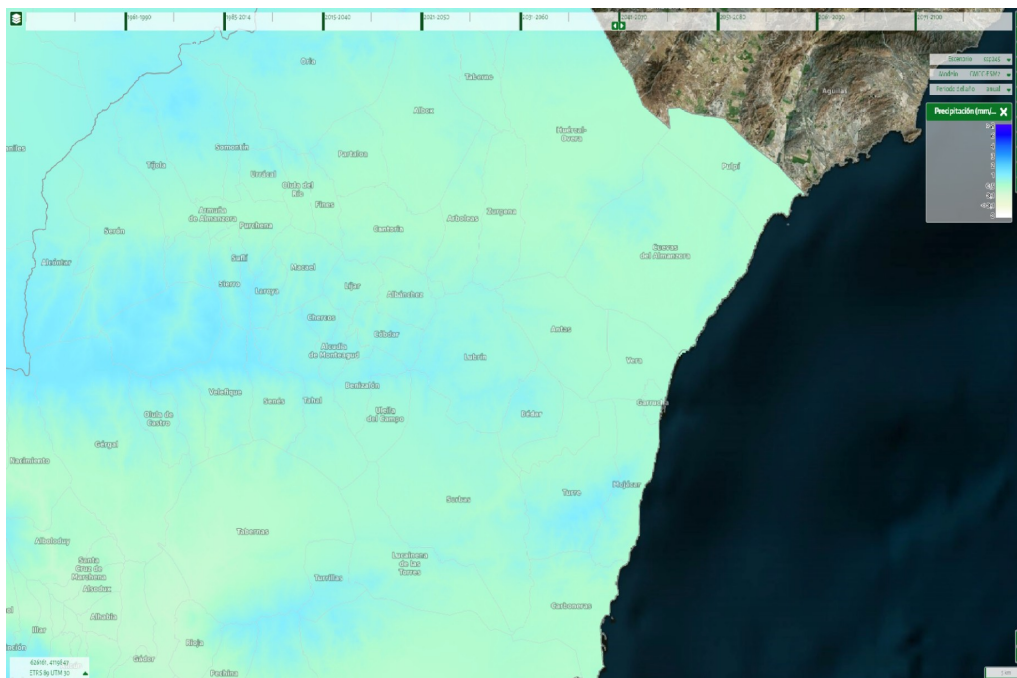
Ilustración 27: Evolución de la precipitación anual en el periodo comparado 2041-2070. Fuente: SICMA
