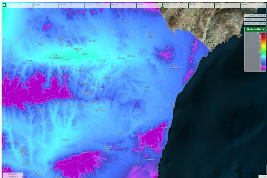
Ilustración 50: Evolución del número de días de calor (40 °C) en el periodo comparado 2041-2070. Fuente: SICMA
