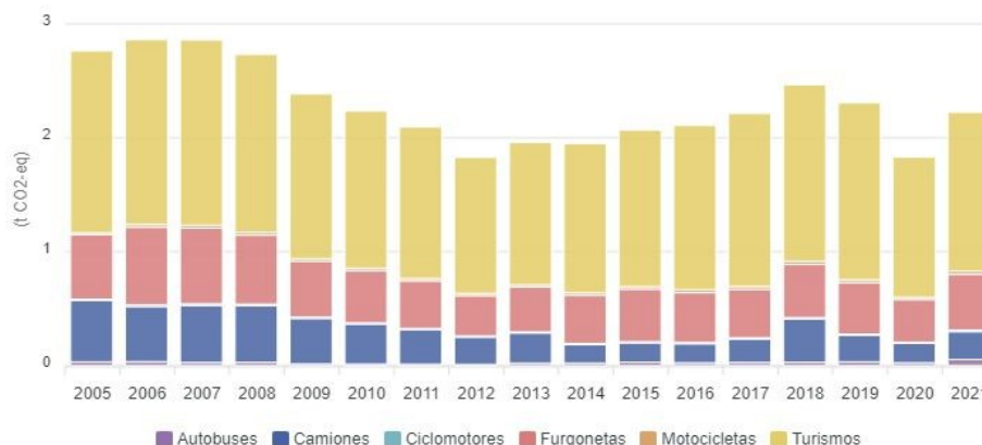
Gráfico 11: Evolución de emisiones GEI per cápita por transporte, por año y tipo de vehículo en Sorbas (2005-2021). Fuente: Huella de Carbono Municipal. Junta de Andalucía.
