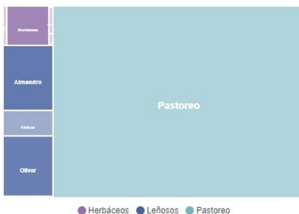
Gráfico 59: Hectáreas y emisiones por tipo de aprovechamiento en Levante III.1 (2021).
