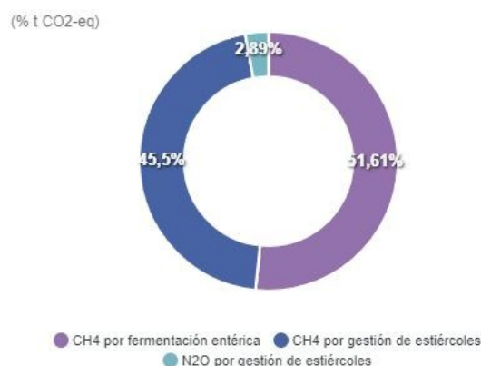
Gráfico 19: Porcentaje según el tipo de emisiones – ganadería en Sorbas (2021). Fuente: Huella de Carbono Municipal. Junta de Andalucía.
