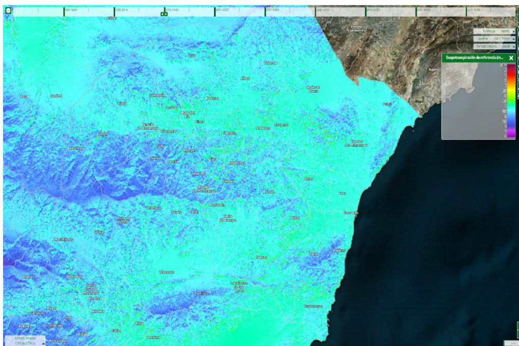
Ilustración 93: Evolución de la evapotranspiración de referencia en el periodo comparado 2015-2040. Fuente: SICMA
