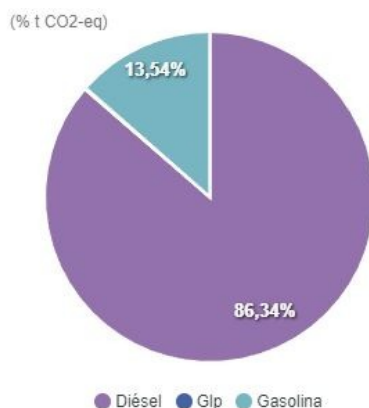
Gráfico 49: Emisiones por tipo de combustible en Levante III.1 (2021). Fuente: Huella de Carbono Municipal. Junta de Andalucía.
