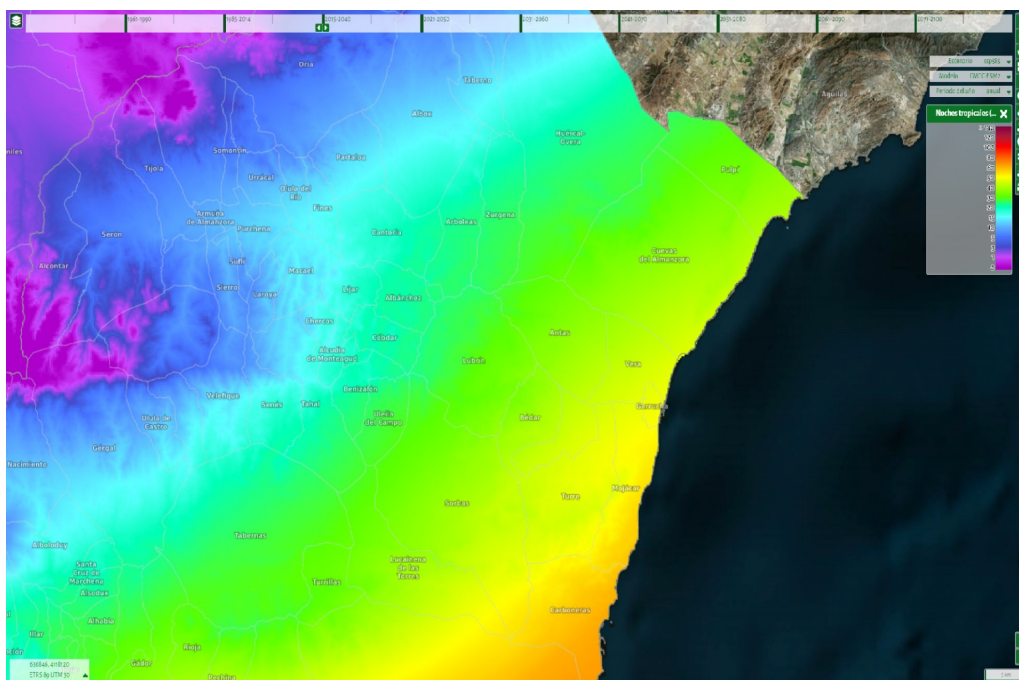
Ilustración 95: Evolución del número de noches tropicales (22 °C) en el periodo comparado 2015-2040. Fuente: SICMA
