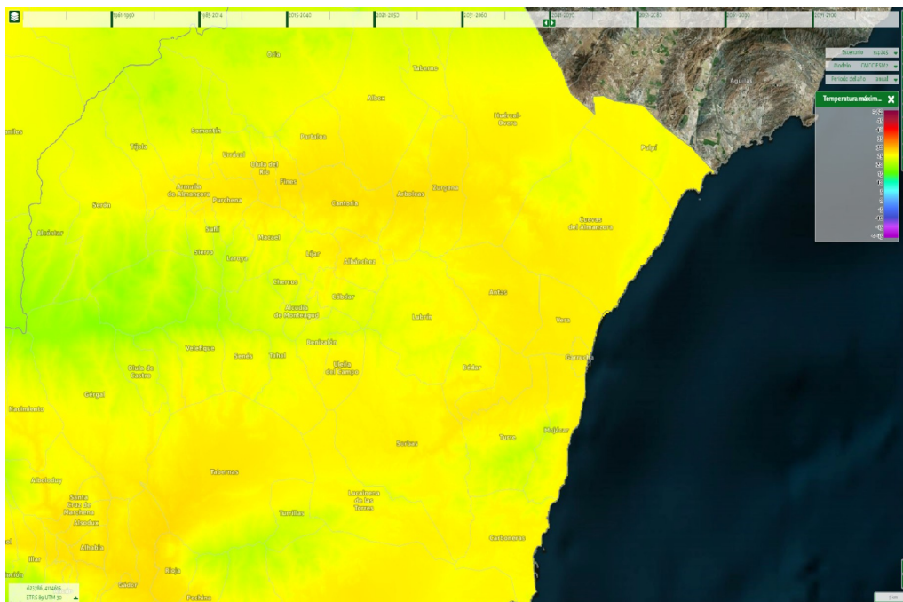
Ilustración 25: Evolución de las temperaturas máximas anuales en el período comparado 2041-2070. Fuente: SICMA
