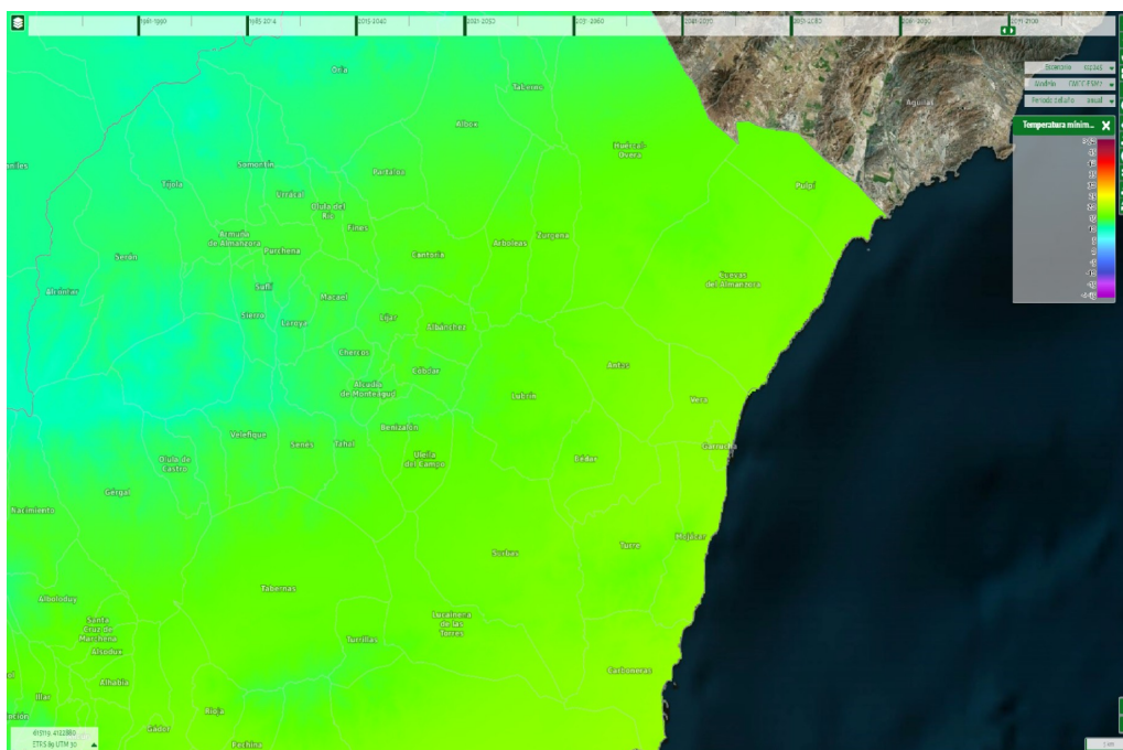
Ilustración 84: Evolución de la temperatura mínima anual en el periodo comparado 2071-2100. Fuente: SICMA
