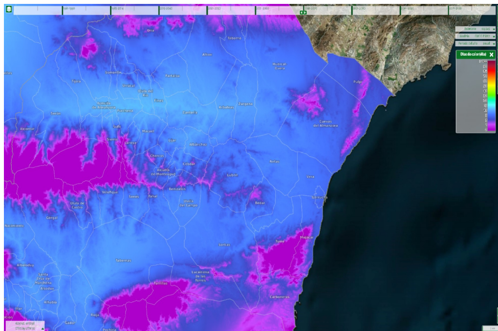
Ilustración 29: Evolución del número de días de calor (40 °C) en el periodo comparado 2041-2070. Fuente: SICMA
