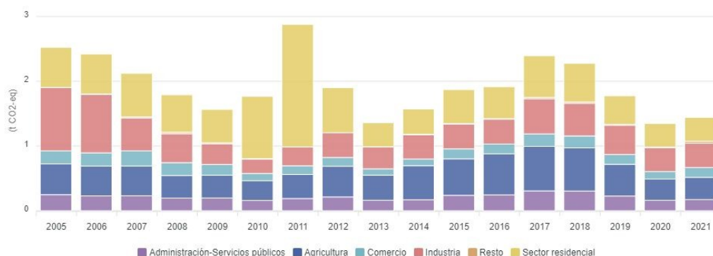
Gráfico 9: Evolución de las emisiones del consumo eléctrico per cápita por año y subsector en Sorbas (2005-2021). Fuente: Huella de Carbono Municipal. Junta de Andalucía.
