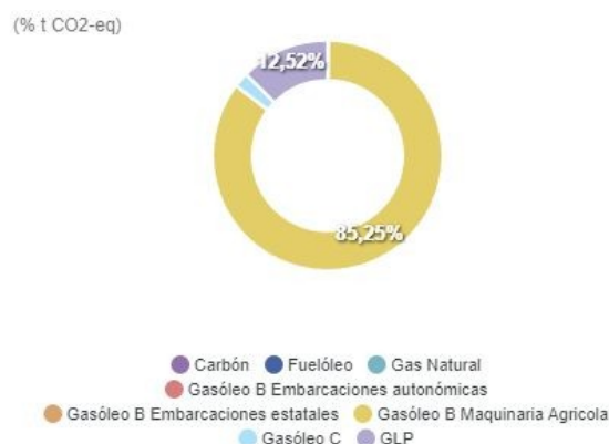
Gráfico 15: Porcentaje de emisiones por tipo de combustible - inst fijas en Sorbas (2021). Fuente: Huella de Carbono Municipal. Junta de Andalucía.
