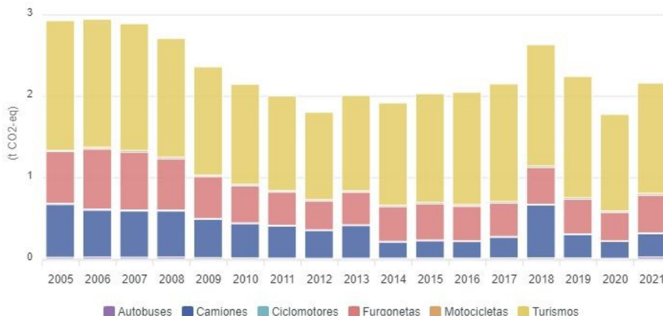
Gráfico 47: Evolución de emisiones GEI per cápita por transporte, por año y tipo de vehículo en Levante III.1 (2005-2021). Fuente: Huella de Carbono Municipal. Junta de Andalucía.
