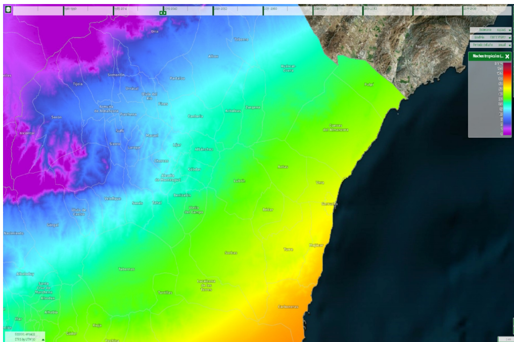
Ilustración 23: Evolución del número de noches tropicales (22 °C) en el periodo comparado 2015-2040. Fuente: SICMA
