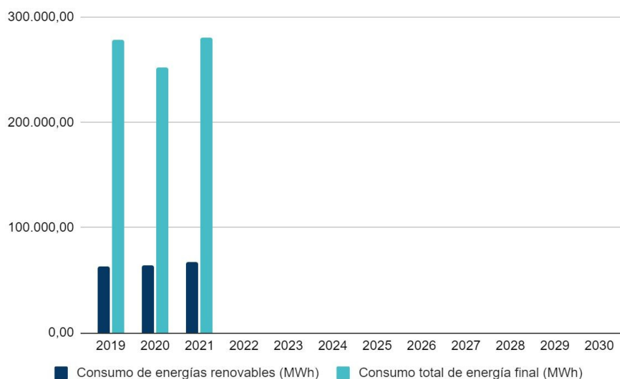
Gráfico 67: Evolución del consumo de energía final y del consumo de energías renovables (Mwh) en Levante III.1 (2019-2030). Fuente: Huella de Carbono Municipal. Junta de Andalucía.
