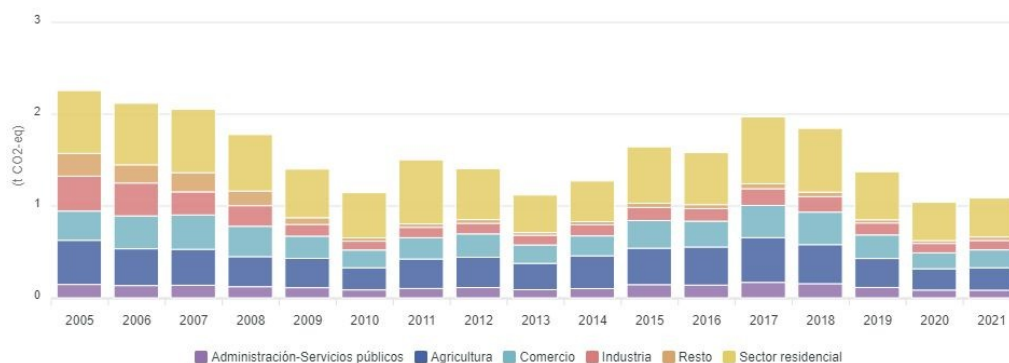
Gráfico 45: Evolución de las emisiones del consumo eléctrico per cápita por año y subsector en Levante III.1. (2005-2021) Fuente: Huella de Carbono Municipal. Junta de Andalucía.
