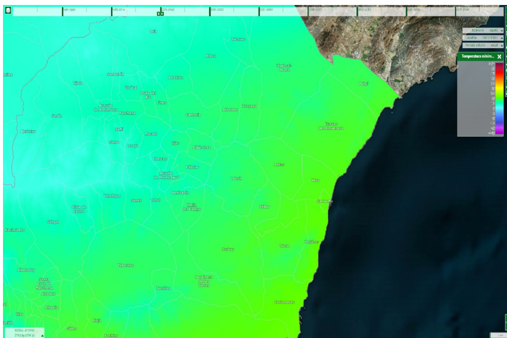
Ilustración 91: Evolución de las temperaturas mínimas anuales en el periodo comparado 2015-2040. Fuente: SICMA
