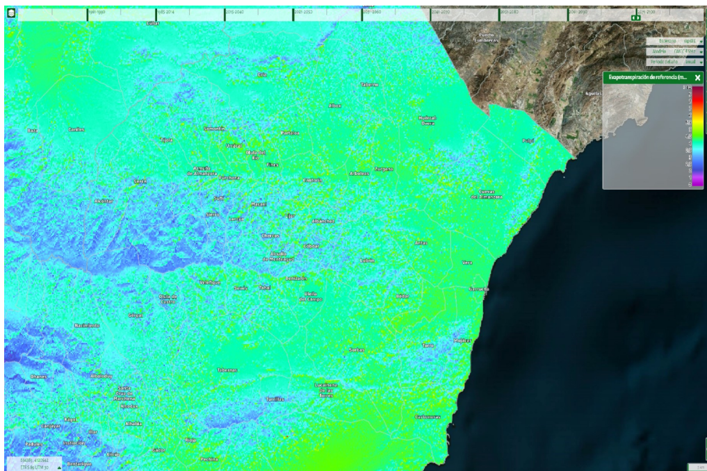
Ilustración 56: Evolución de la Evapotranspiración de referencia en el periodo comparado 2071-2100. Fuente: SICMA
