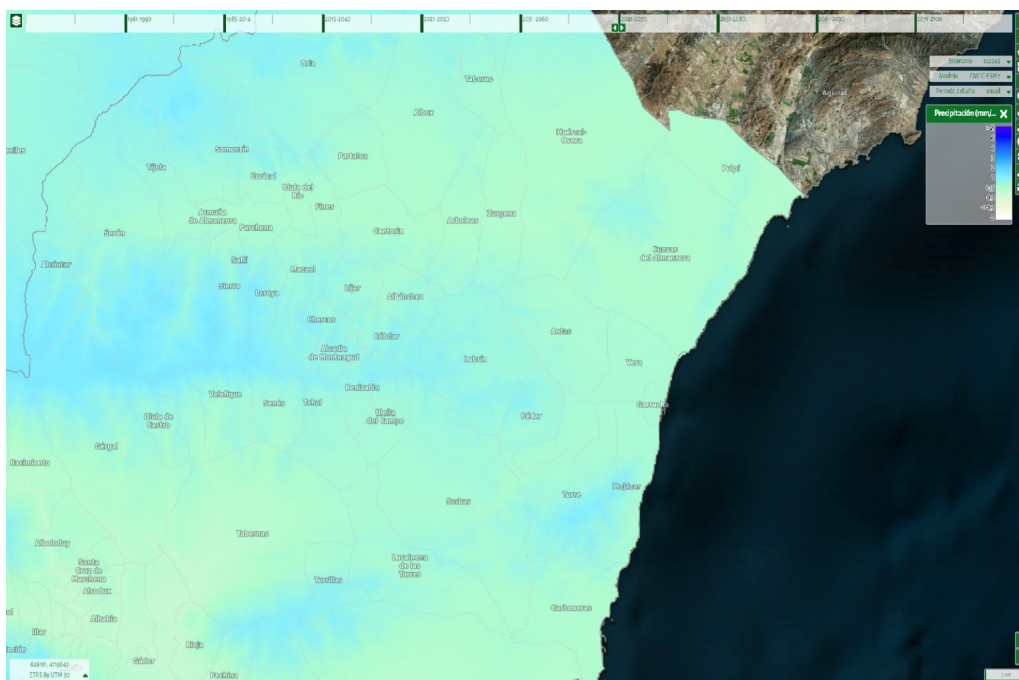
Ilustración 78: Evolución de la precipitación anual en el periodo comparado 2041-2070. Fuente: SICMA
