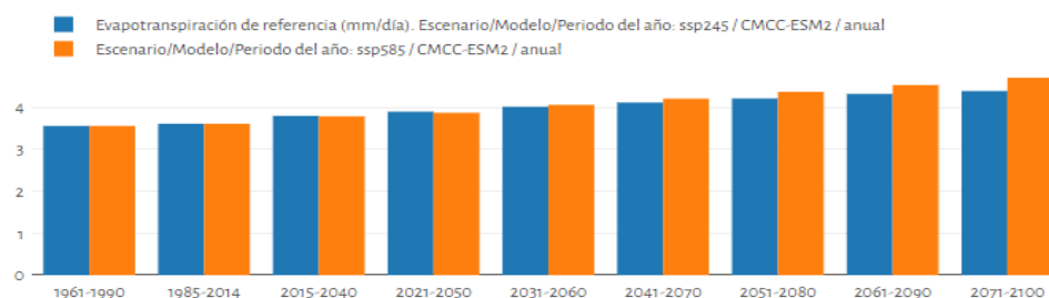
Ilustración 14: Evolución de la evapotranspiración de referencia anual en los diferentes periodos.
