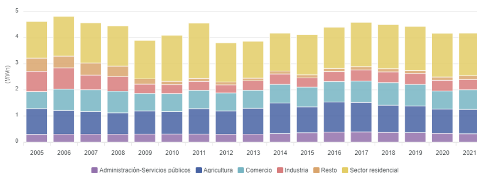
Gráfico 62: Evolución consumo eléctrico per cápita por subsectores en Levante III.1 (2005-2021).
