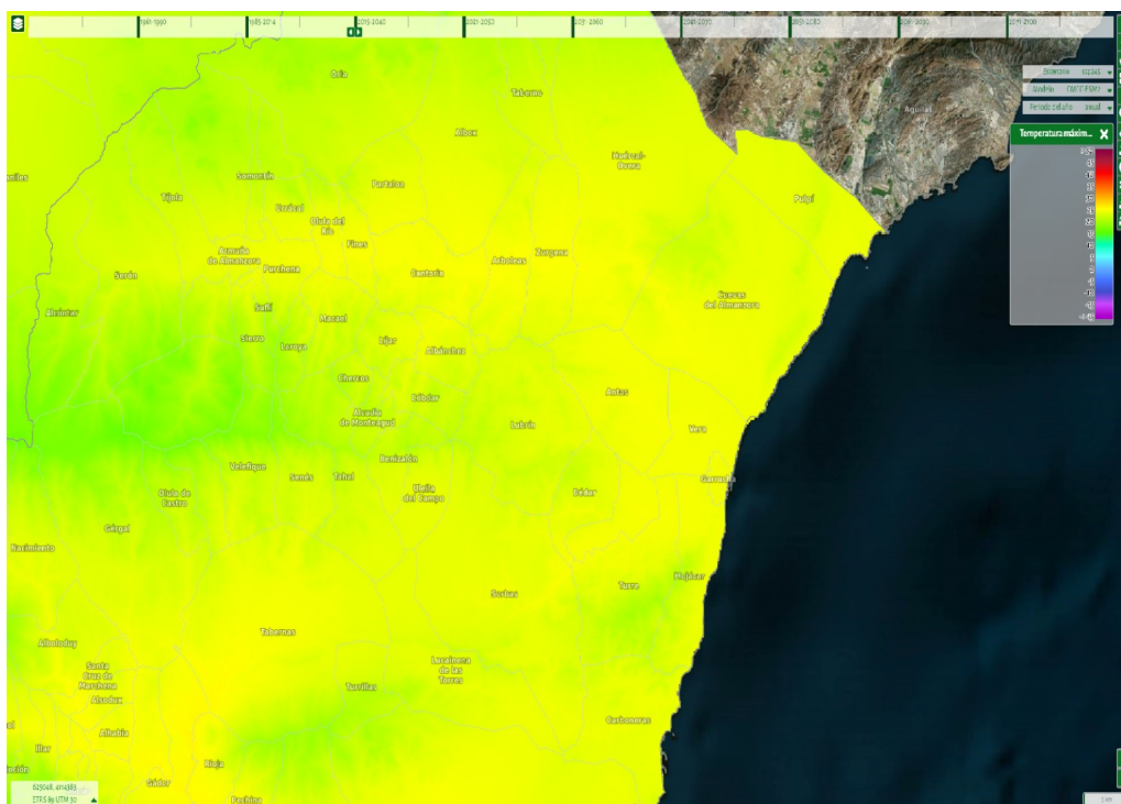
Ilustración 69: Evolución de las temperaturas máxima anual en el periodo comparado 1980-2040.
