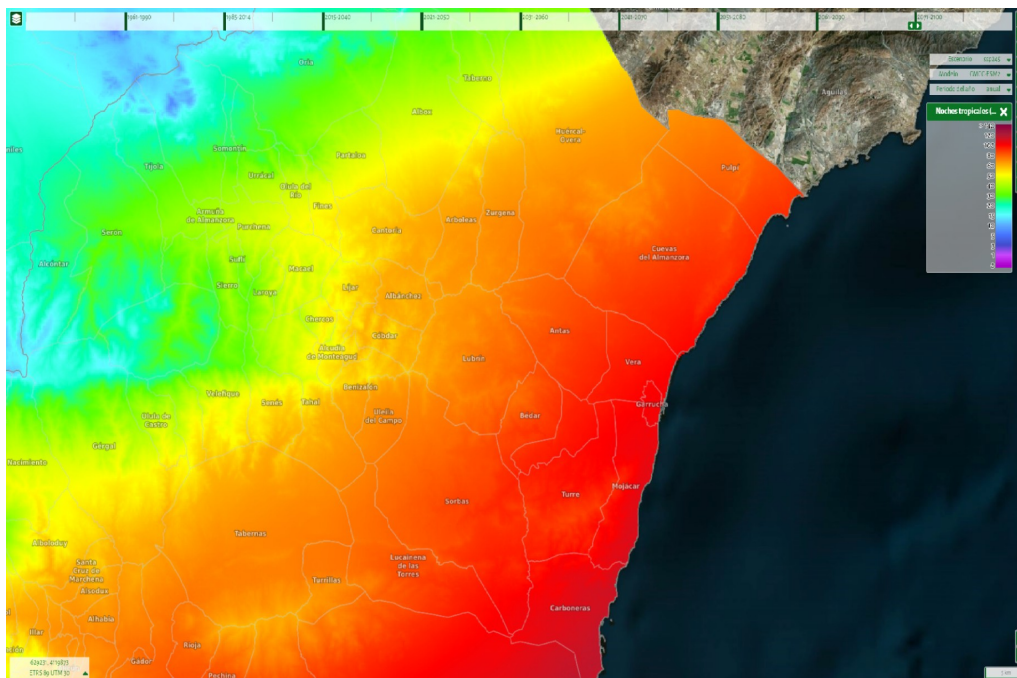
Ilustración 37: Evolución del número de noches tropicales (22 °C) anual en el periodo comparado 2071-2100. Fuente: SICMA
