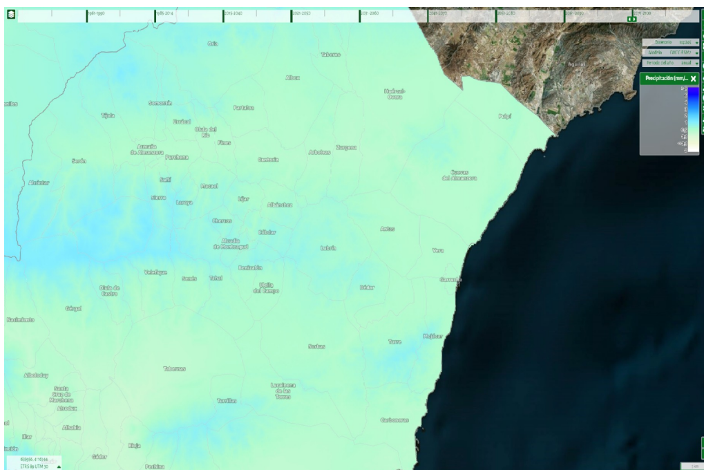
Ilustración 85: Evolución de la precipitación anual en el periodo comparado 2071-2100. Fuente: SICMA
