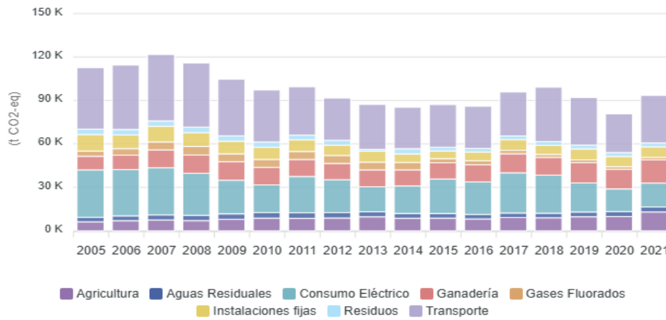
Gráfico 42: Evolución de emisiones GEI, por año y sector en Levante III.1 (2005-2021). Fuente: Huella de Carbono Municipal. Junta de Andalucía.
