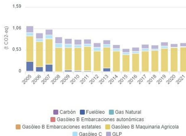
Gráfico 14: Evolución de emisiones GEI per cápita por año y tipo de combustible - inst fijas en Sorbas (2005-2021). Fuente: Huella de Carbono Municipal. Junta de Andalucía.
