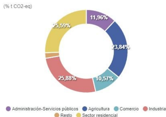
Gráfico 10: Porcentaje de emisiones por consumo eléctrico por subsectores en Sorbas (2021). Fuente: Huella de Carbono Municipal. Junta de Andalucía.
