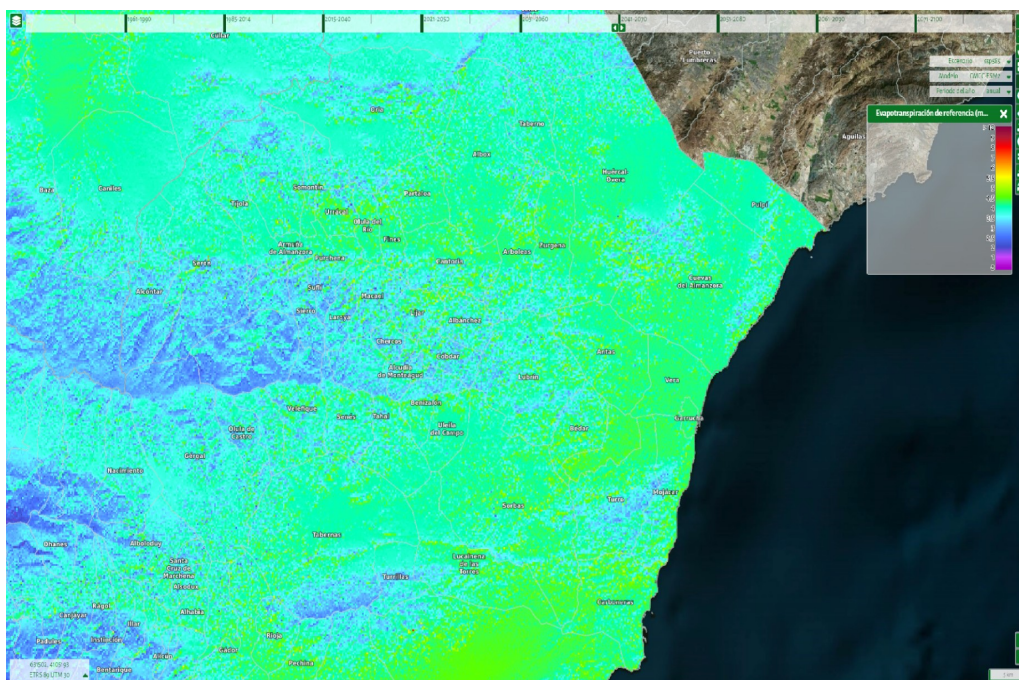
Ilustración 100: Evolución de la Evapotranspiración de referencia en el periodo comparado 2041-2070. Fuente: SICMA
