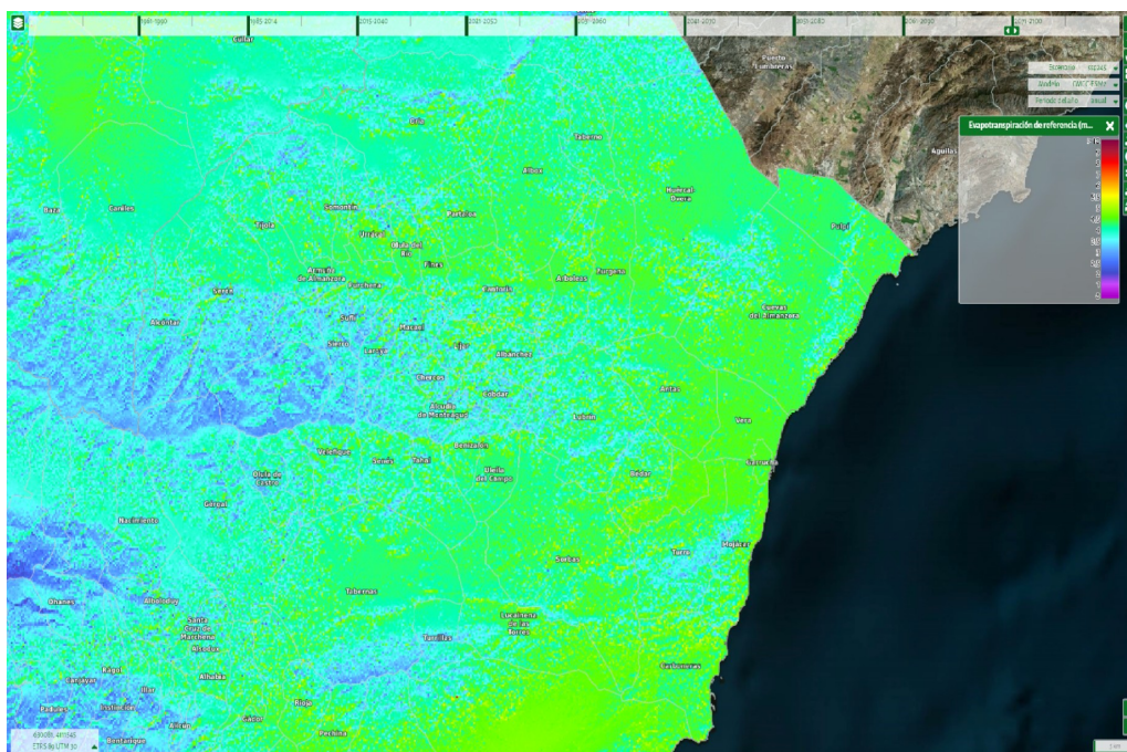
Ilustración 86: Evolución de la evapotranspiración de referencia en el periodo comparado 2071-2100. Fuente: SICMA
