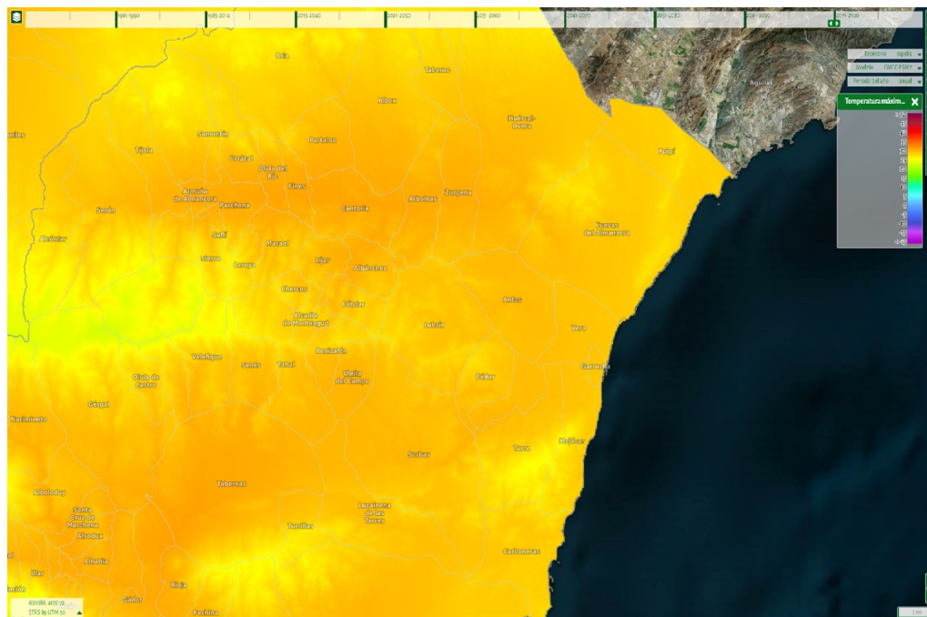
Ilustración 53: Evolución de las temperaturas máxima anual en el periodo comparado 2071-2100. Fuente: SICMA
