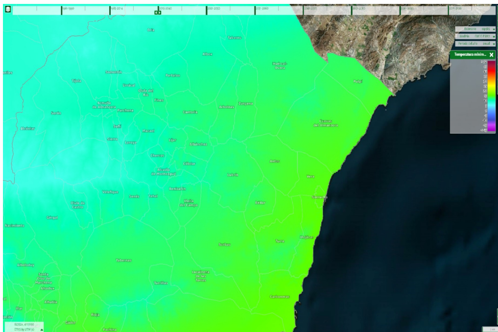
Ilustración 40: Evolución de las temperaturas mínimas anuales en el periodo comparado 2015-2040. Fuente: SICMA
