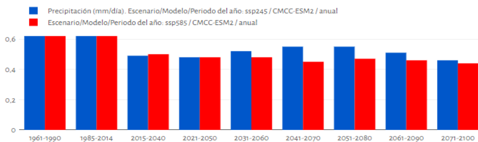
Ilustración 13: Evolución de las precipitaciones anuales en los diferentes periodos.
