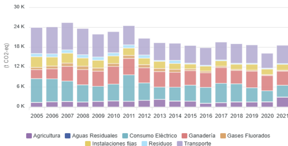
Gráfico 6: Evolución de emisiones GEI, por año y sector en Sorbas (2005-2021). Fuente: Huella de Carbono Municipal. Junta de Andalucía.
