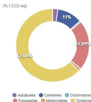
Gráfico 12: Porcentaje de emisiones por tipo de vehículo en Sorbas (2021). Fuente: Huella de Carbono Municipal. Junta de Andalucía.
