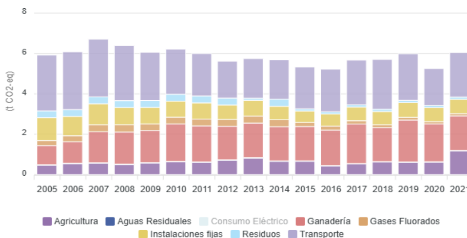
Gráfico 8: Evolución de emisiones difusas GEI per cápita, por año y sector en Sorbas (2005-2021). Fuente: Huella de Carbono Municipal. Junta de Andalucía.
