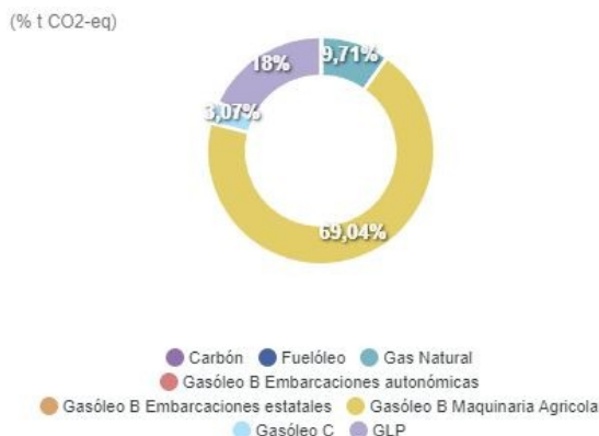
Gráfico 51: Porcentaje de emisiones por tipo de combustible - inst fijas en Levante III.1 (2021). Fuente: Huella de Carbono Municipal. Junta de Andalucía.
