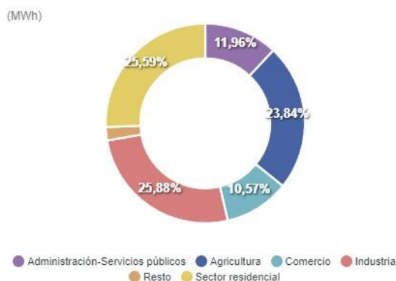
Gráfico 27: Consumo eléctrico por subsectores en Sorbas (2021).
