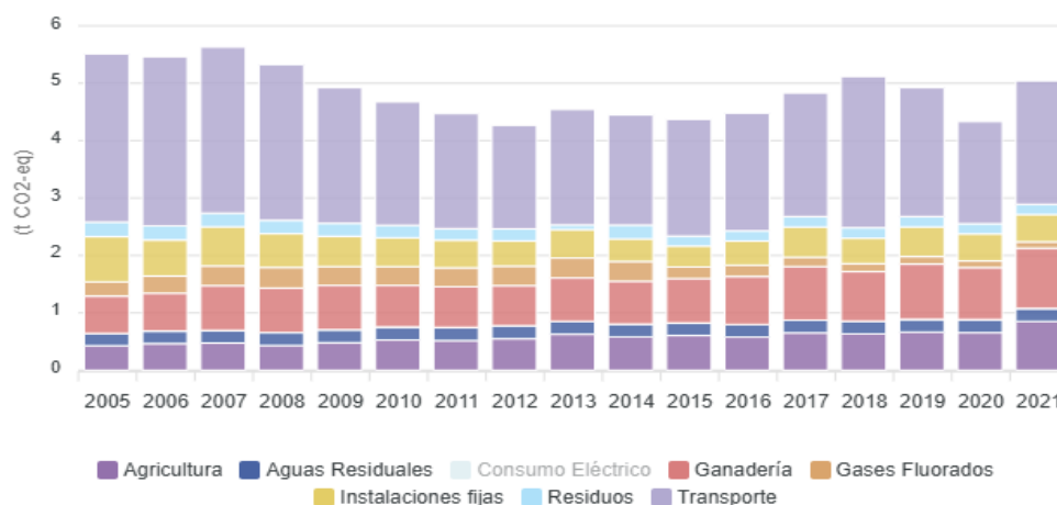
Gráfico 44: Evolución de emisiones difusas GEI per cápita, por año y sector en Levante III.1 (2005-2021). Fuente: Huella de Carbono Municipal. Junta de Andalucía.
