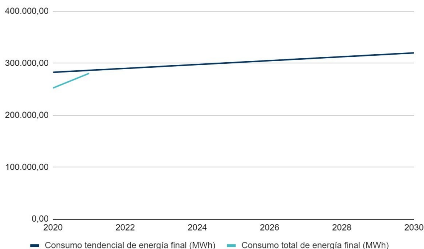
Gráfico 66: Evolución del consumo tendencial y del consumo de energía final (Mwh) en Levante III.1 (2020-2030). Fuente: Huella de Carbono Municipal. Junta de Andalucía.
