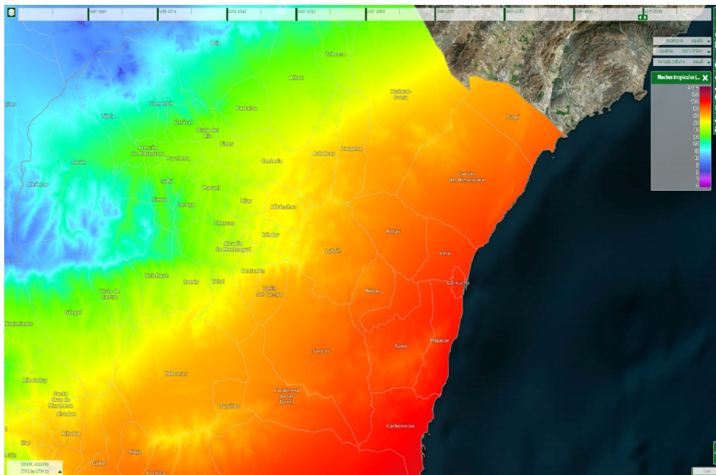
Ilustración 109: Evolución del número de noches tropicales (22 °C) anual en el periodo comparado 2071-2100. Fuente: SICMA
