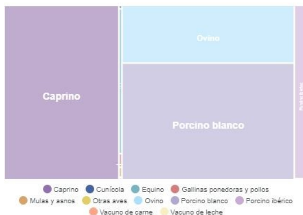
Gráfico 20: Número de cabezas y emisiones por categoría de ganado en Sorbas (2021). Fuente: Huella de Carbono Municipal. Junta de Andalucía.
