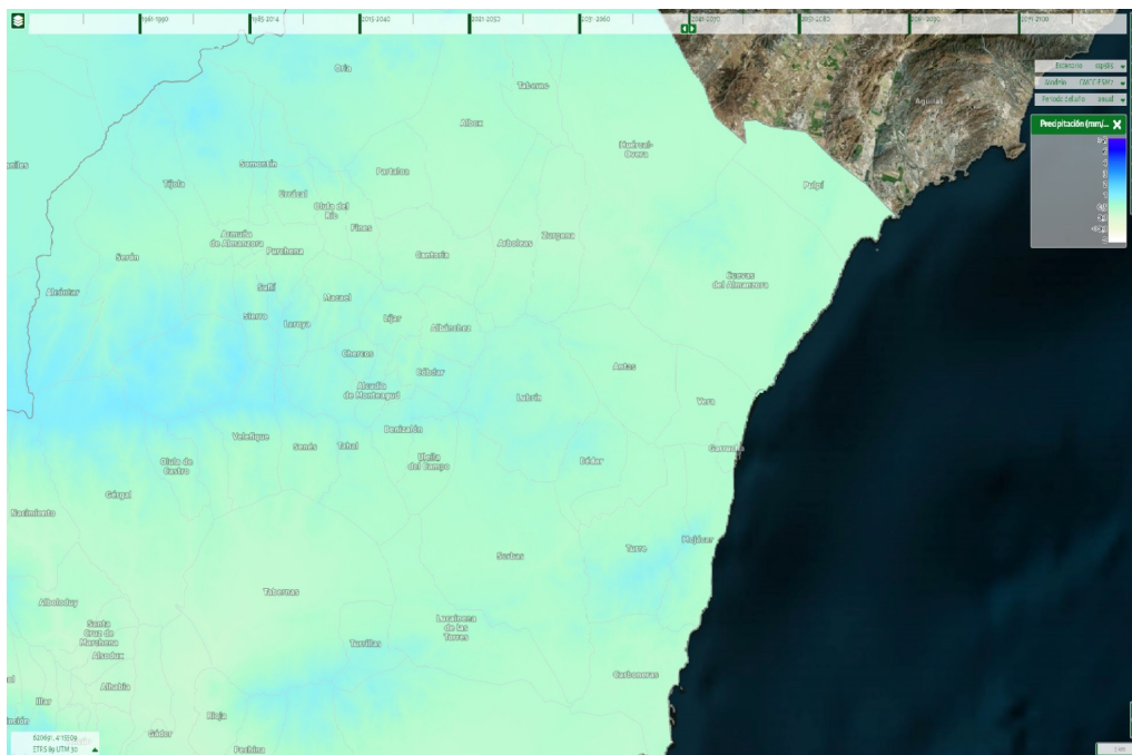
Ilustración 48: Evolución de la precipitación anual en el periodo comparado 2041-2070. Fuente: SICMA
