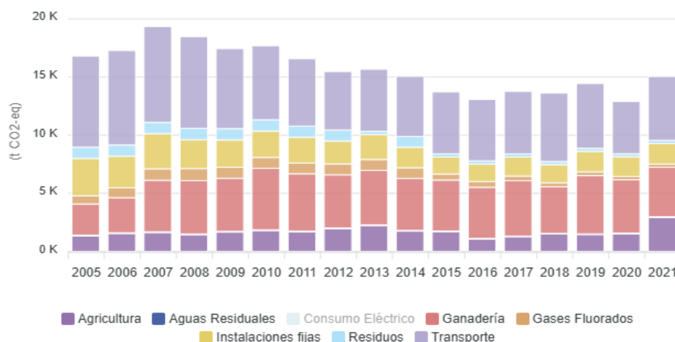
Gráfico 7: Evolución de emisiones difusas, por año y sector en Sorbas (2005-2021). Fuente: Huella de Carbono Municipal. Junta de Andalucía.
