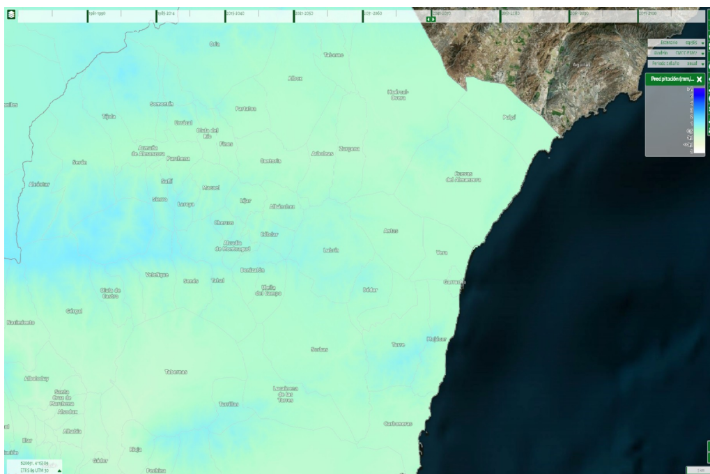
Ilustración 99: Evolución de la precipitación anual en el periodo comparado 2041-2070. Fuente: SICMA
