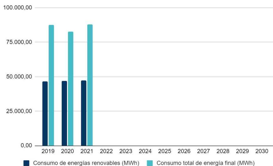
Gráfico 31: Evolución del consumo de energía final y del consumo de energías renovables (Mwh) en Sorbas (2020-2030).
