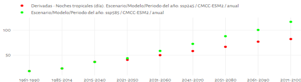
Ilustración 16: Evolución de las noches tropicales anuales en los diferentes periodos.
