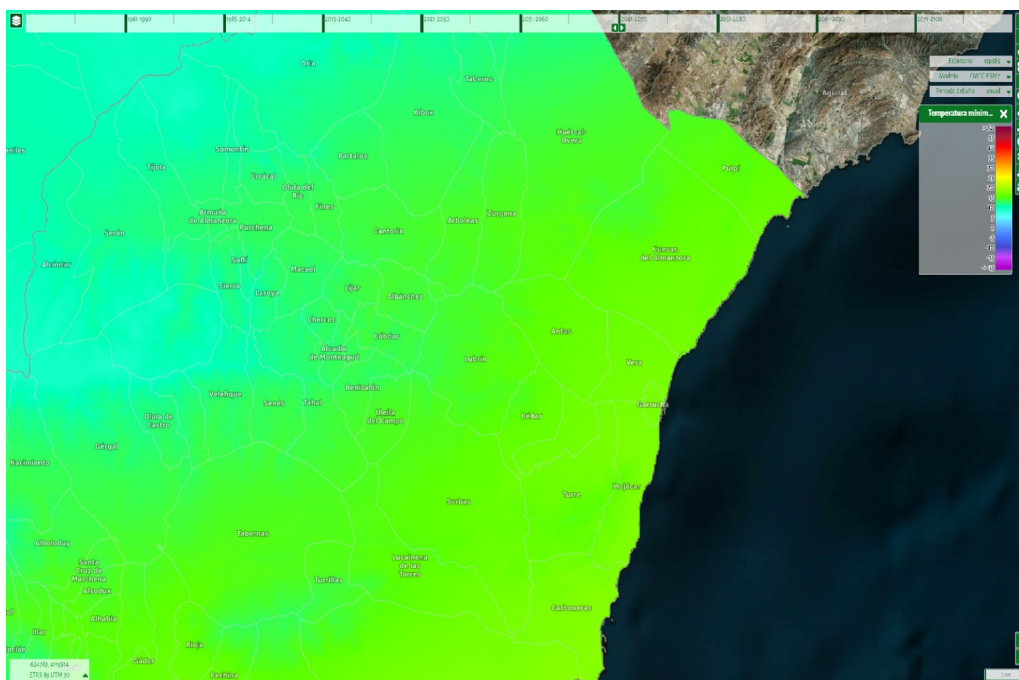
Ilustración 98: Evolución de las temperaturas mínimas anuales en el periodo comparado 2041-2070. Fuente: SICMA
