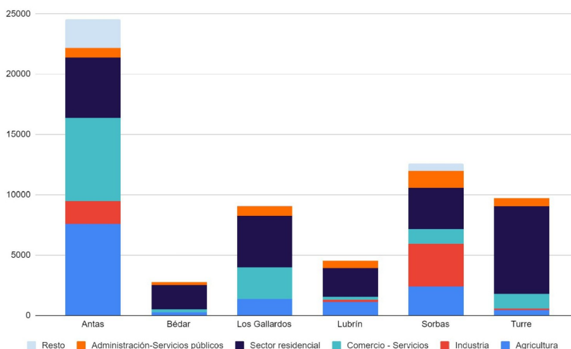
Gráfico 38: Consumo de energía eléctrica por sectores en Levante (III.1.). Fuente: E.P. a partir de los datos del Sistema de Información Multiterritorial de Andalucía (SIMA), 2022.
