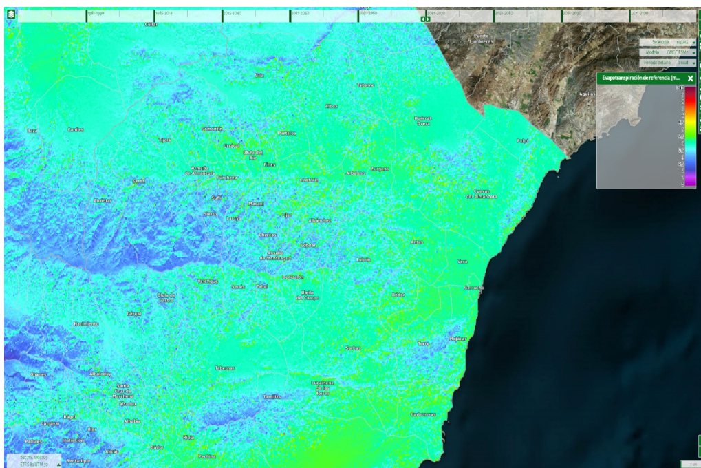
Ilustración 79: Evolución de la evapotranspiración anual en el periodo comparado 2041-2070. Fuente: SICMA
